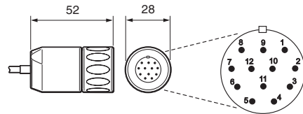
12针圆形插头 (端子代码V)
