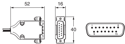
15针D型插头 (端子代码L)
