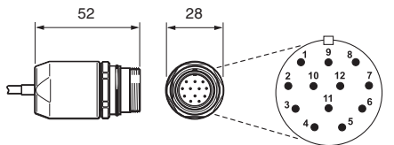
12针圆形连接器插头 (端子代码W)
