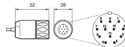
12针圆形插头（端子代码R）
